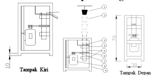
Gambar 3.1 Rancangan mesin pemotong ring limbah cup minuman
