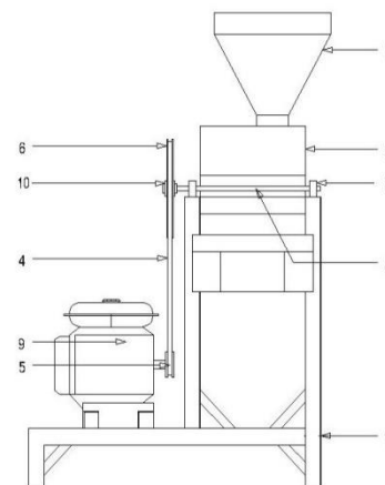
Gambar 2.2 Gambar mesin yang direncanakan
