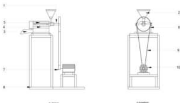
Gambar 3.1 Konstruksi mesin Pengupas Kulit Ari Biji Kopi
