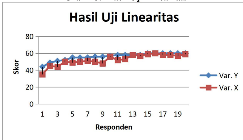
Grafik 5. Hasil Uji Linearitas
