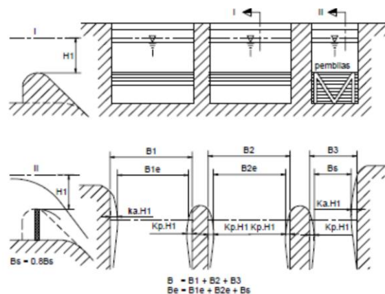
Gambar 1. Lebar Efektif Bendung
