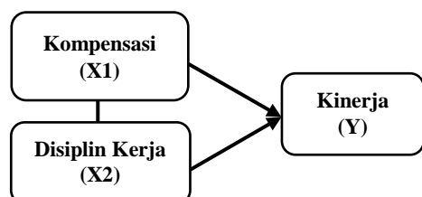
Gambar 2. 1 Kerangka Pemikiran
